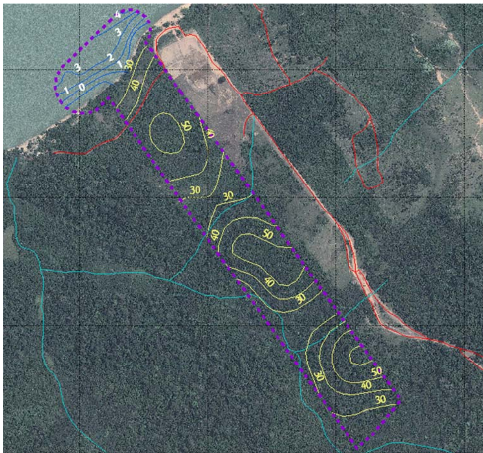
Figura 48. Batimetria da AID.
