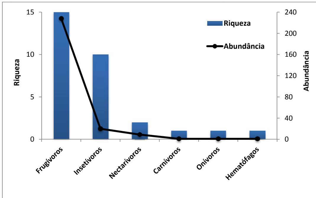
Gráfico 30. A fauna de morcegos da ETC Rurópolis dividida por guildas alimentar.
