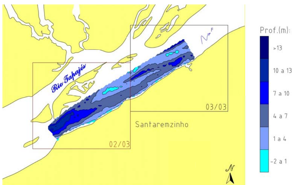
Figura 47. Resultado do levantamento batimétrico.
