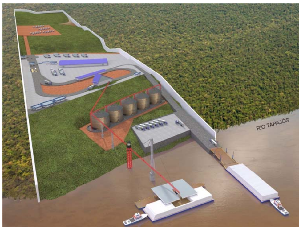
Figura 12. Layout do projeto conceitual da ETC Rurópolis.
