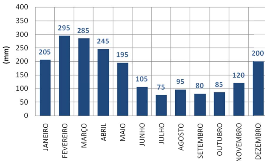
Gráfico 1. Precipitação acumulada em Itaituba – PA (INMET).
